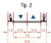
PRESJEK B __ B
