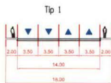
PROFILI PLANIRANIH SAOBRAĆAJNICA
